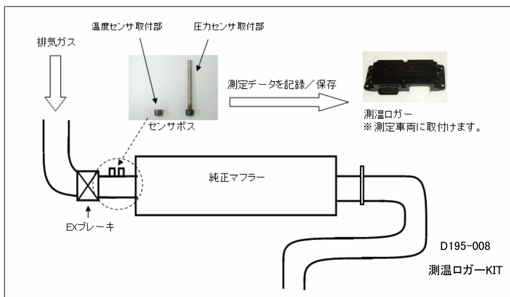
測温イメージ
