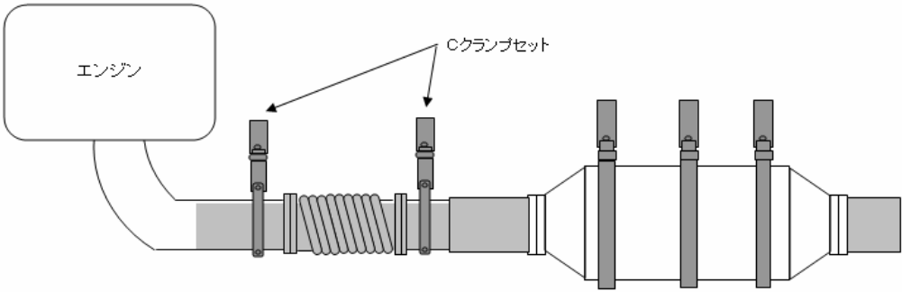
取付け例
