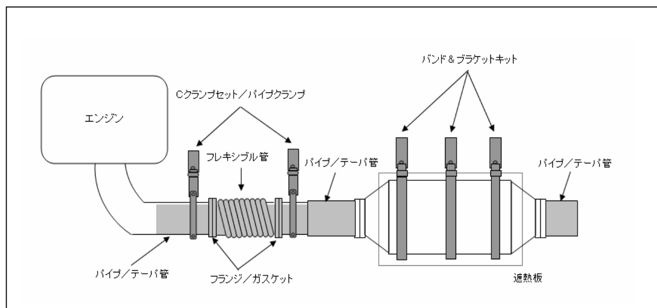
オプション部品使用例
