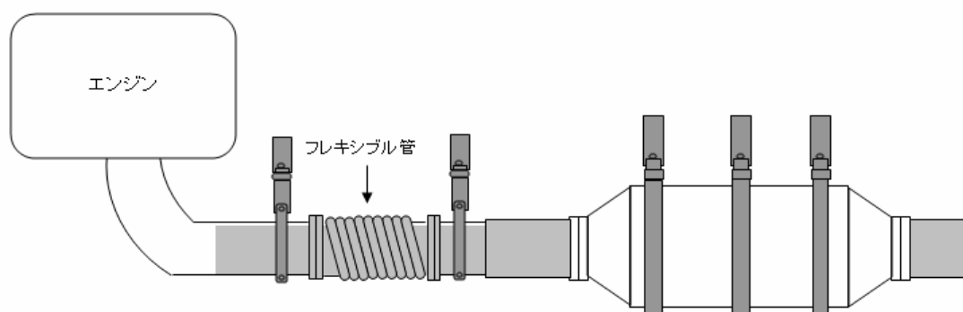
取付け例
